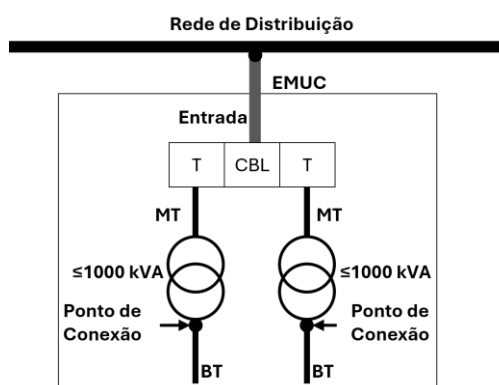
Figura 10 – CT até 2000 kVA, (somente BT e MT)
